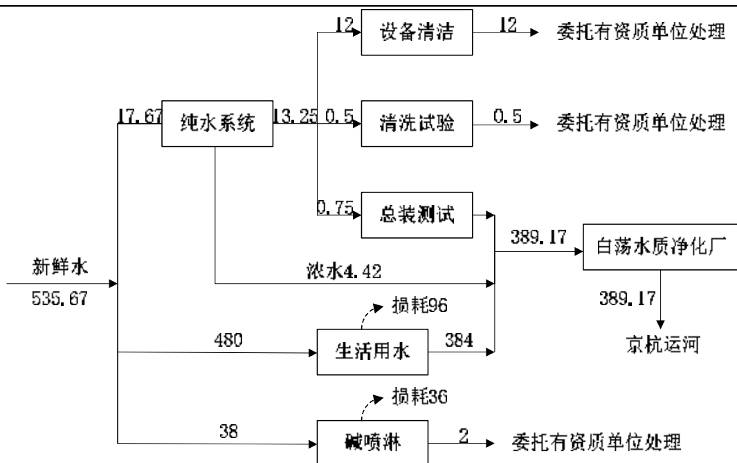
图 2-6 现有项目水平衡图 (单位 t/a)
