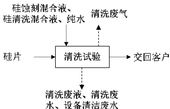
图 2-5 现有项目清洗试验工艺流程图
