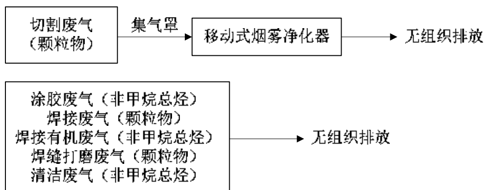
图 4-1 废气收集处理工艺流程图
