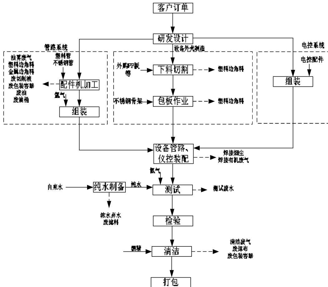
图 2-4 现有项目生产工艺流程图
