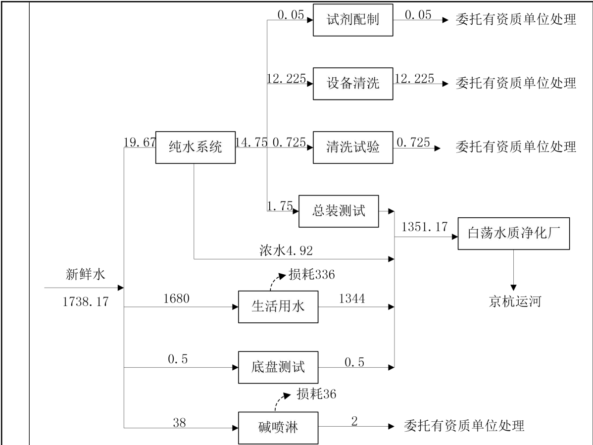
图 2-2 本次技改后石林路厂区水平衡图 (t/a)
